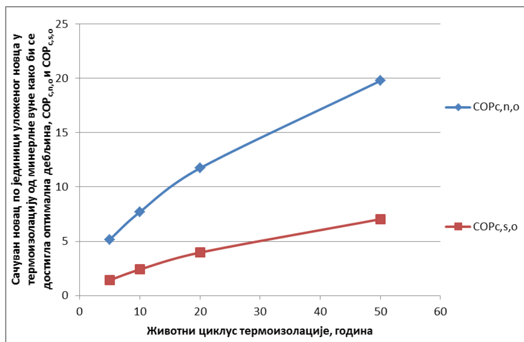
Слика 11.19. Уштеда новца по јединици уложеног новца у термоизолацију до оптималне дебљине када се као материјал користи минерална вуна
