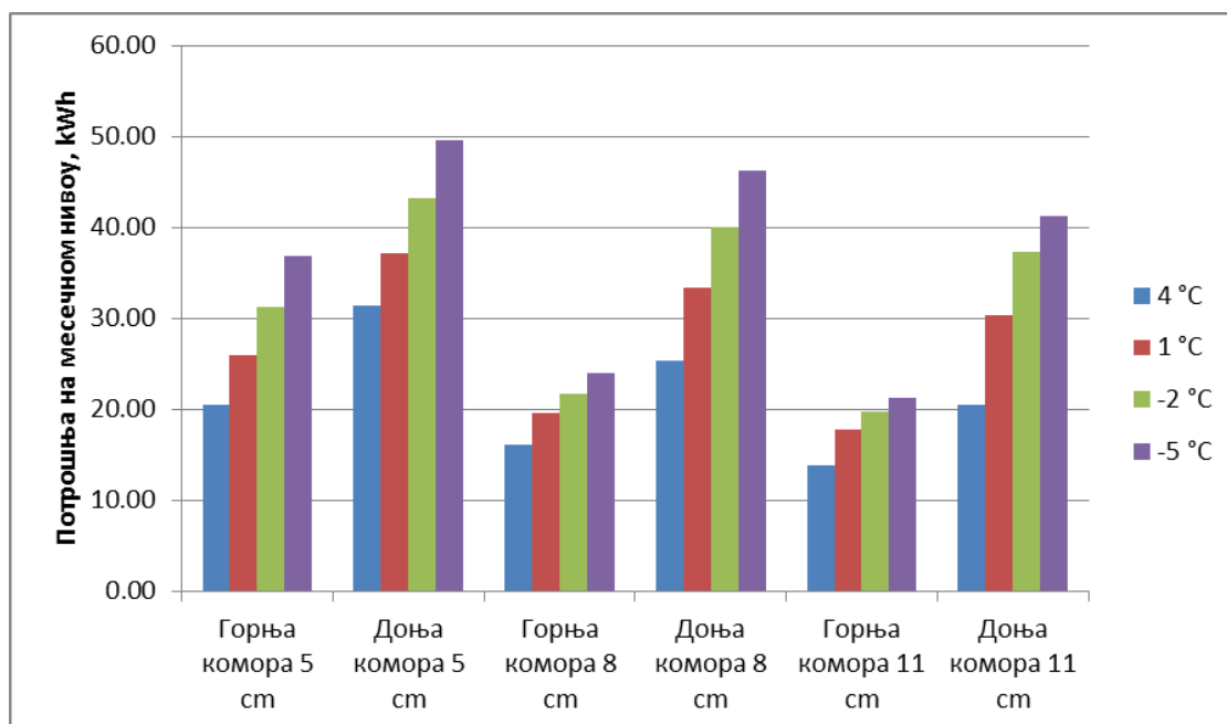
Слика 9.24. Потрошња на месечном нивоу за све дебљине термоизолационог слоја при различитим температурама спољашње средине
