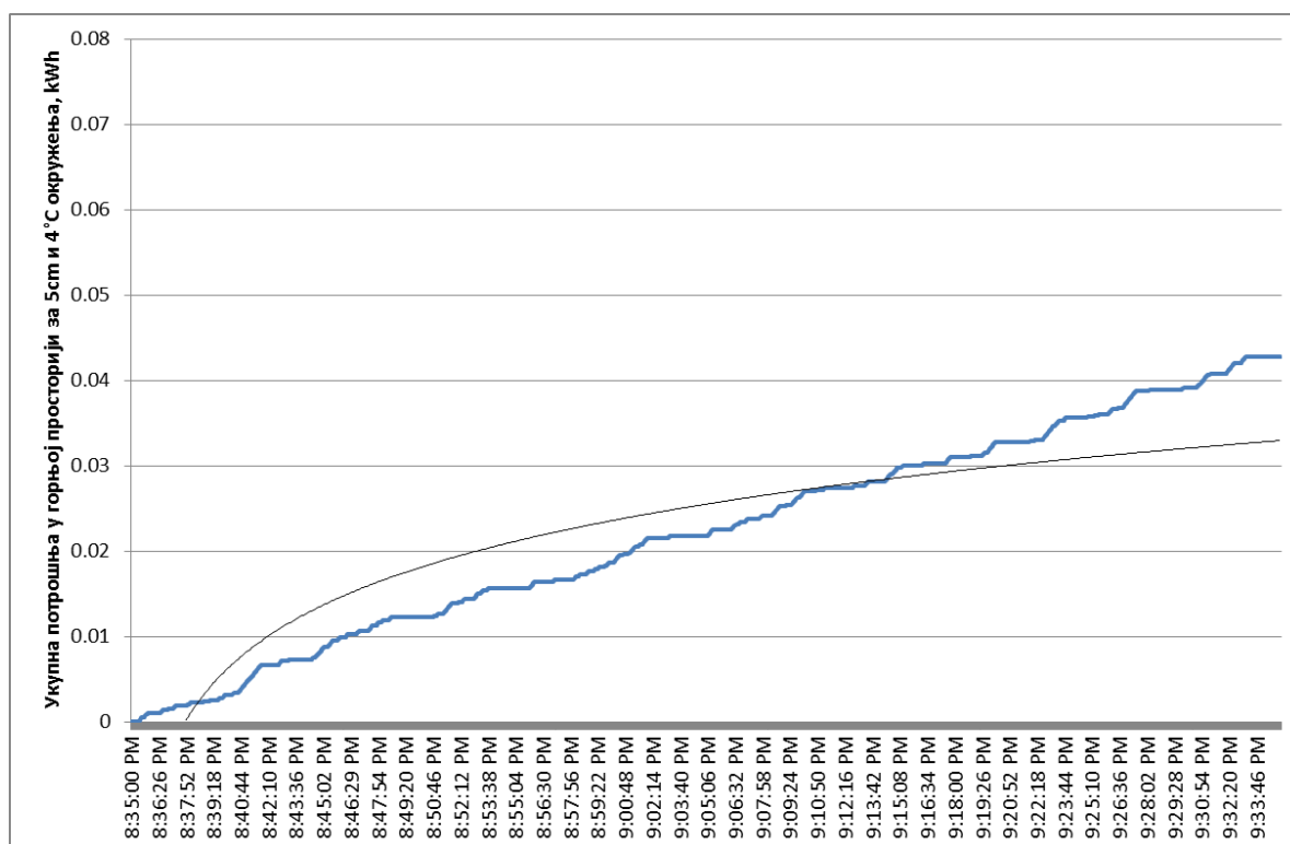
Слика 9.22. Укупна потрошња енергије у горњој комори при температури од 4°C и дебљини термоизолације од 5 ст
