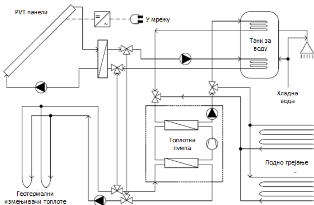
Слика 2.6. Шематски приказ система хибридни фотонапонски панели на кући у Холандији [22]
