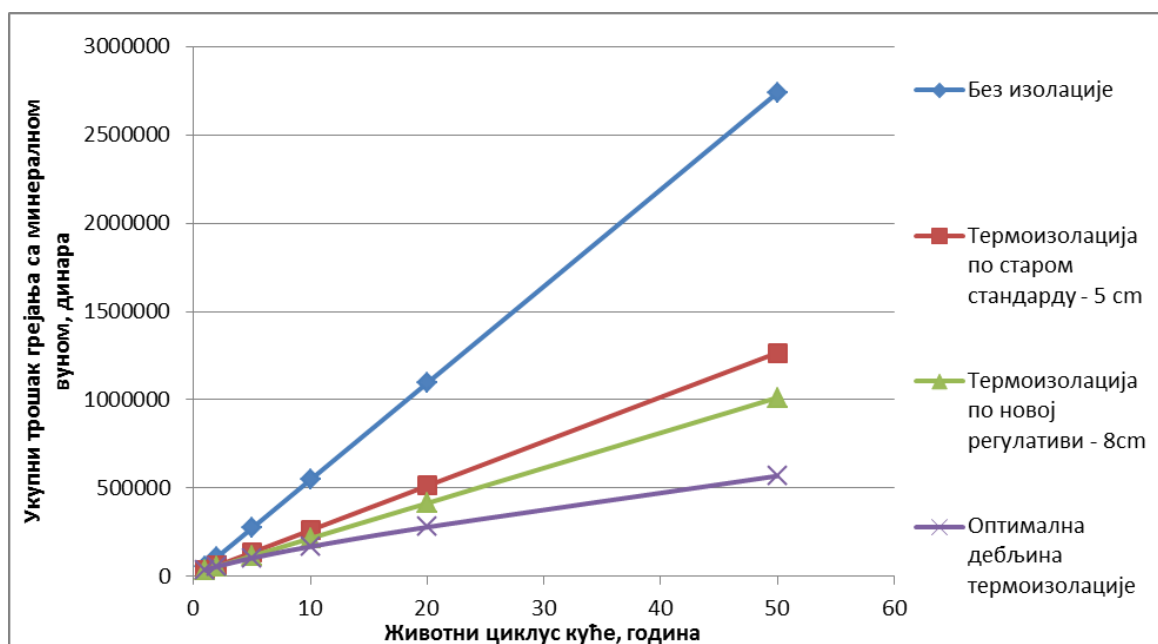
Слика 11.17. Укупна трошак грејања у зависности од животног циклуса. Линеје представљају куће без изолације, са изолацијом по старом стандарду, са изолацијом по новој регулативи, и са изолацијом оптималне дебљине. Термоизолациони материјал је минерална вуна.
