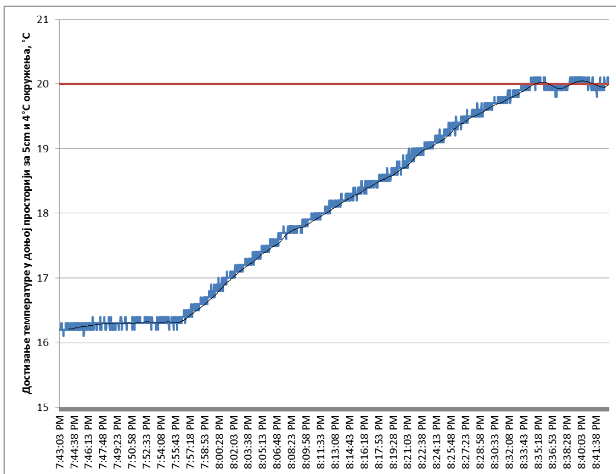
Слика 9.14. Достигање температуре на почетку мерења у доњој комори при температури од 4°C и дебљини термоизолације од 5 cm
