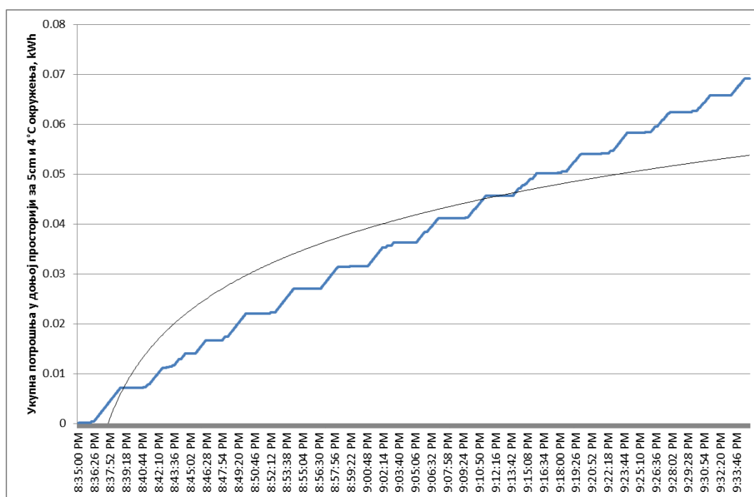
Слика 9.18. Укупна потрошња енергије у доњој комори при температури од 4°C и дебљини термоизолације од 5 cm
