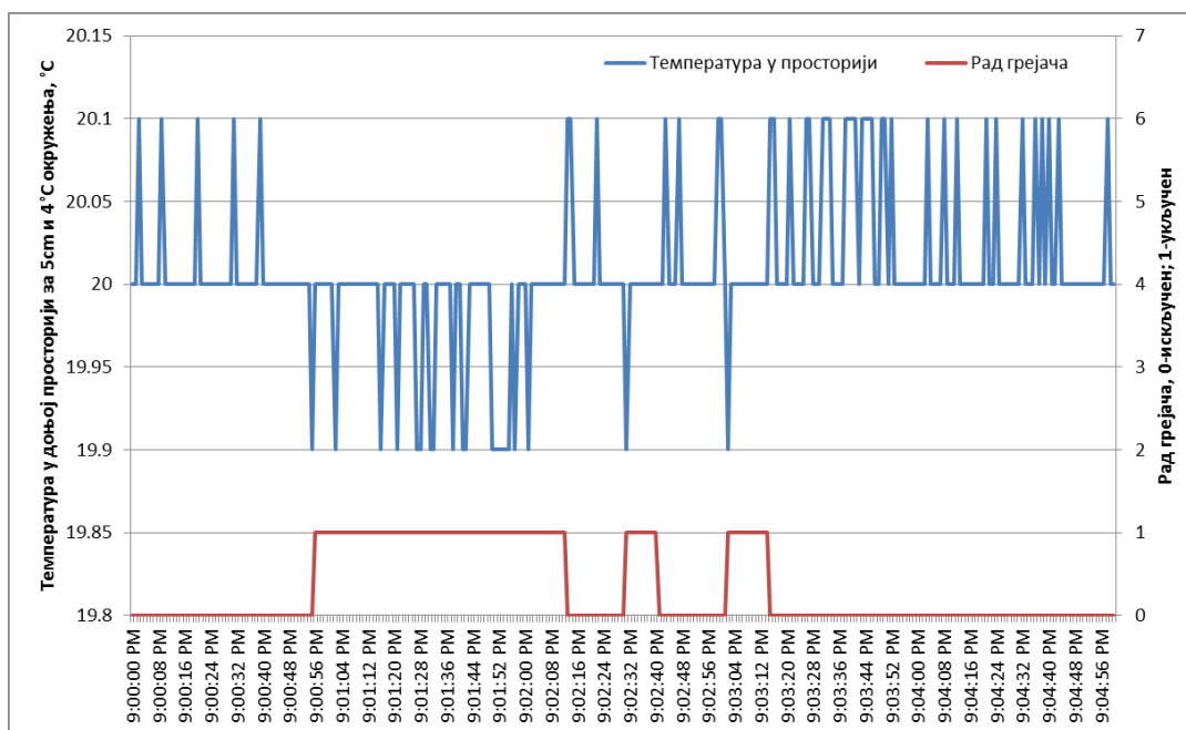
Слика 9.17. Укључивање и искључивање грејача у зависности од унутрашње температуре у доњој комори при спољној температури од 4°C и дебљини термоизолације од 5 cm
