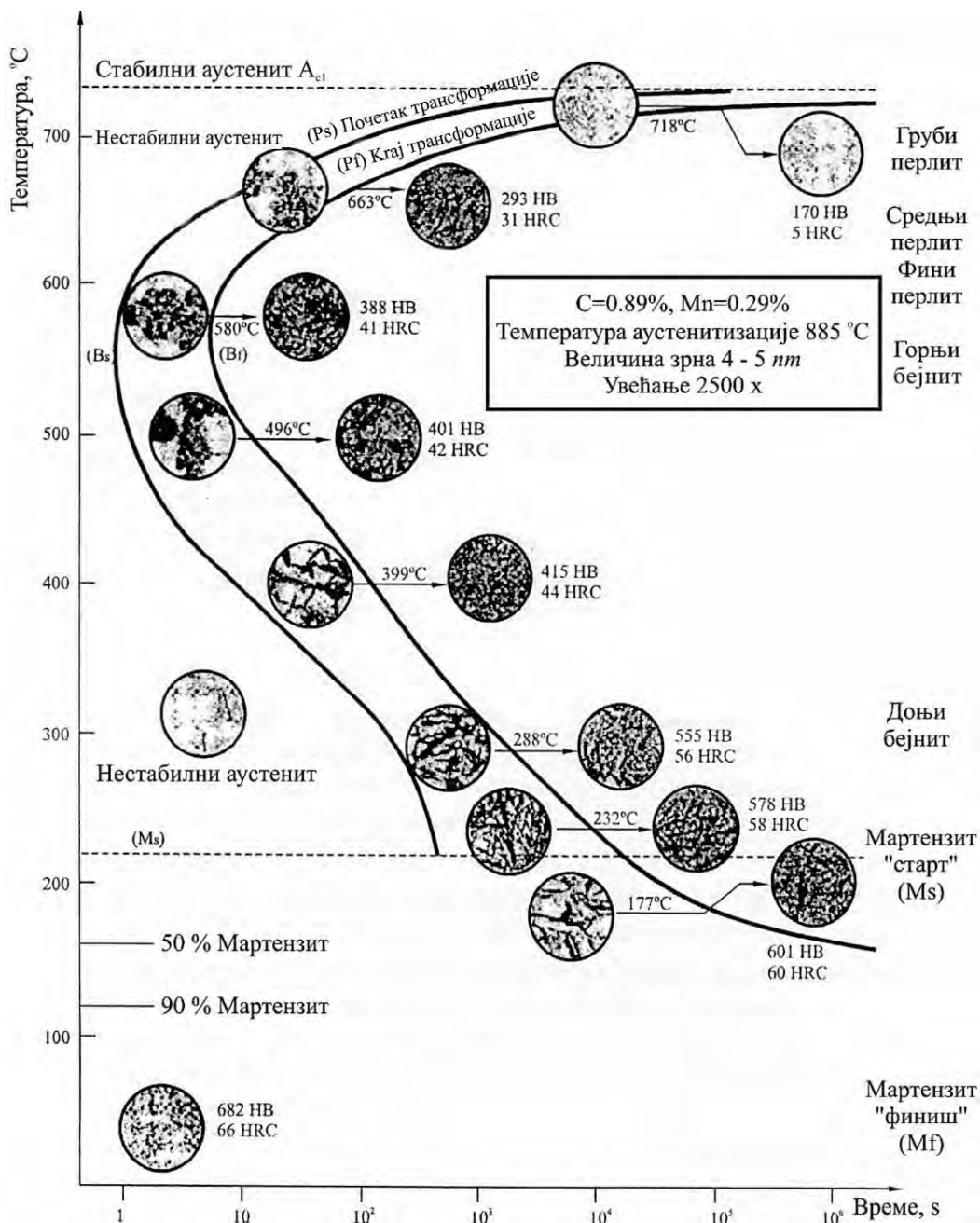
Слика 6.2 Дијаграм изотермичком преображаја аустенита еутектоидног нелегираниог челика (IRA – дијаграм) [97,141,157]
