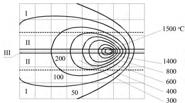
Слика 8.2 Температурско поље око покретног извора топлоте [63,97,141]
