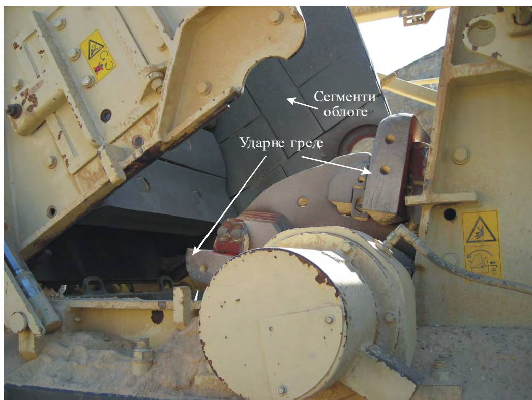
Слика 9.6.20 Унутрашњи изглед ротационе дробилице са ударним гредама капацитета 350 \text{ m}^3/\text{h}
