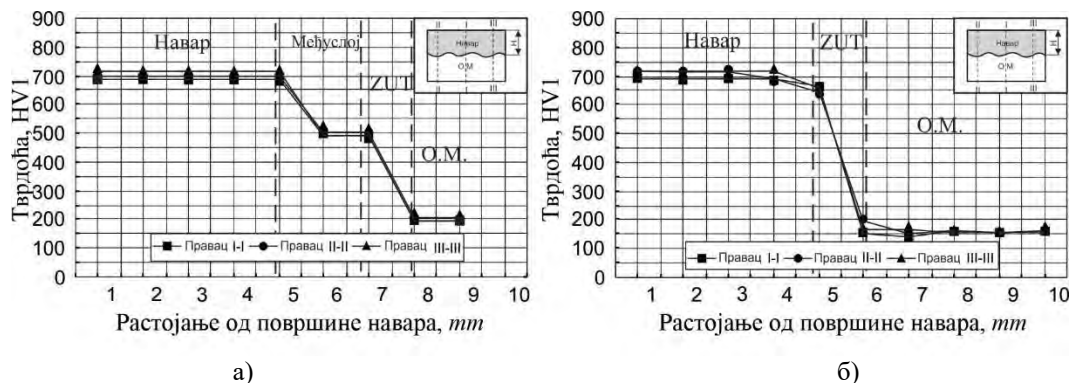
Слика 9.4.16 Распореда тврдоће код блокава припремљених за триболошка испитивања: а) О.М.-Č0363, D.M. међуслоја - FILTUB 12 В, D.M. навара - FILTUB DUR 16, б) О.М. – Č0363, D.M. навара – FILTUB DUR 16
