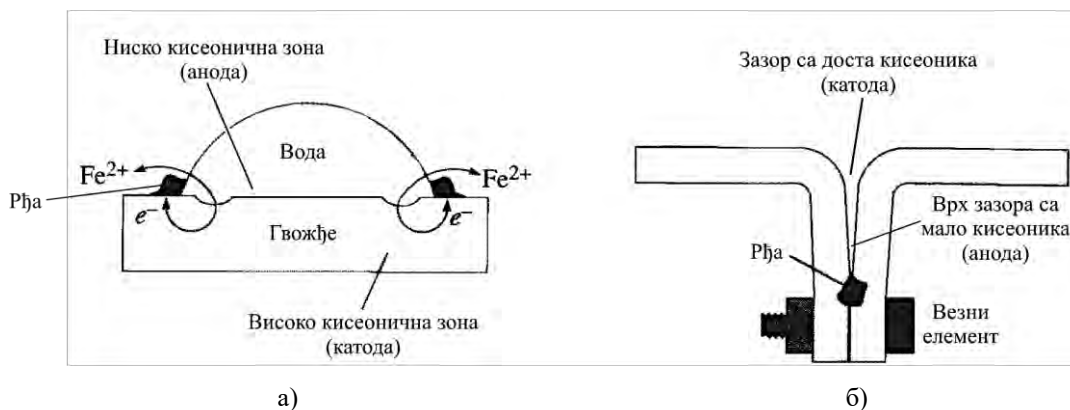
Слика 1.16 Концентрациона ћелија: (а) корозија испод водене капљице на челичној плочи због ниске концентрације кисеоника у води; (б) корозија на врху расцепа због ограниченог приступа кисеоника [7]
