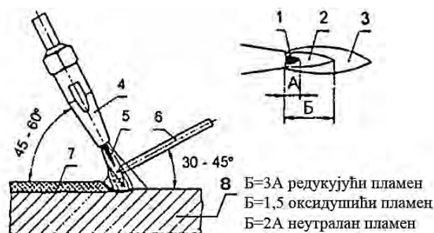
Слика 2.8 Схема гасног наваривања жицом и шипком и препоручено регулисање окси-ацетиленског пламена: 1-језгро, 2-редукујућа зона, 3-оксидишућа зона, 4-гасни горионик, 5-гасни пламен, 6-додатни материјал, 7-навар, 8-основни материјал [63,141]
