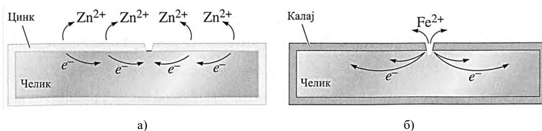
Слика 1.18 Заштитне металне превлаке за челик: а) метална превлака од цинка, б) метална превлака од калаја [7]
