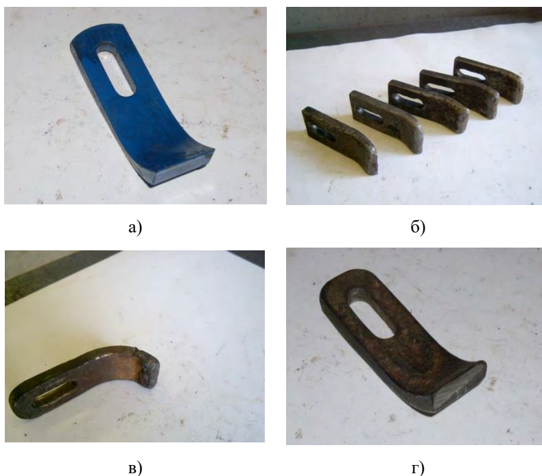
Слика 9.6.30 Изглед ножева уређаја за чишћење растиња: а) нов нож, б) похабани ножеви, в) наварен нож, г) наоштрен нож
