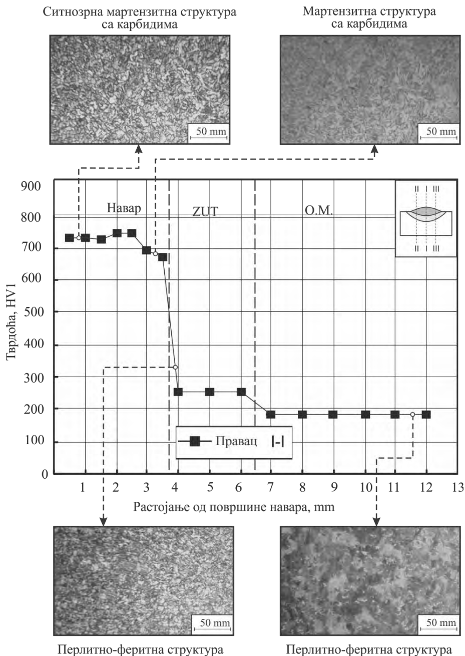
Слика 9.3.31 Микроструктура карактеристичних зона навареног споја: O.M. – \text{S0645} ; D.M. навара - \text{FILTUB DUR 16}
