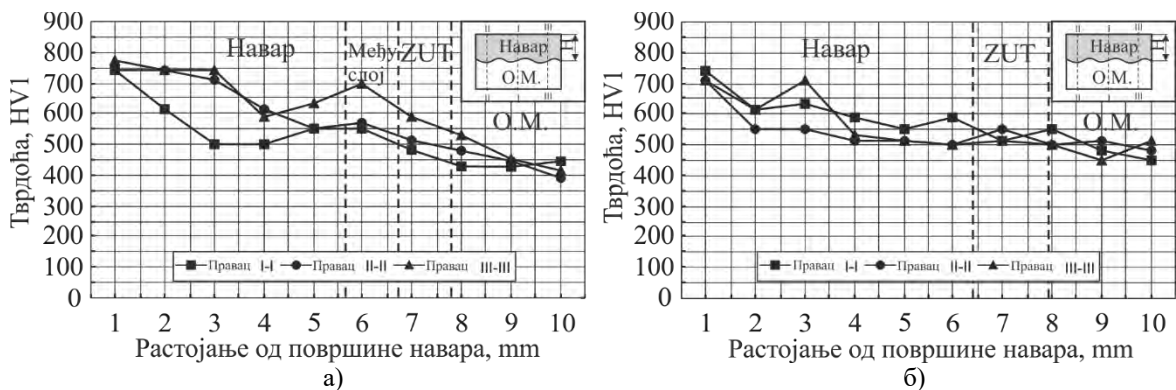
Слика 9.4.10 Расподела тврдоће код блокова припремљених за триболошка испитивања: а) О.М. - ČL3134, D.M. међуслоја - INOX B 18/8/6, D.M. наvara - ABRADUR 58; б) О.М. - ČL3134, D.M. наvara - ABRADUR 58
