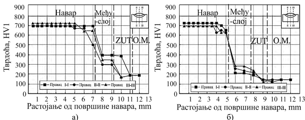
Слика 9.3.14 Распдела тврдоће по пресеку навара: а) O.M. - Č0363; D.M. међуслоја – FILTUB 12 B; D.M. навара - FILTUB DUR 16; б) O.M. – Č0645; D.M. међуслоја – FILTUB 12 B; D.M. навара - FILTUB DUR 16
