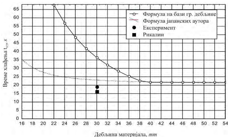
Слика 9.5.11 Упоредни резултати времена хлађења t_{8/5} за Ć1430 дебљине s = 30 mm, при наваривању: T_p = 97 °C, d_e = 5 mm, q_1 = 38667 J/cm [97]
