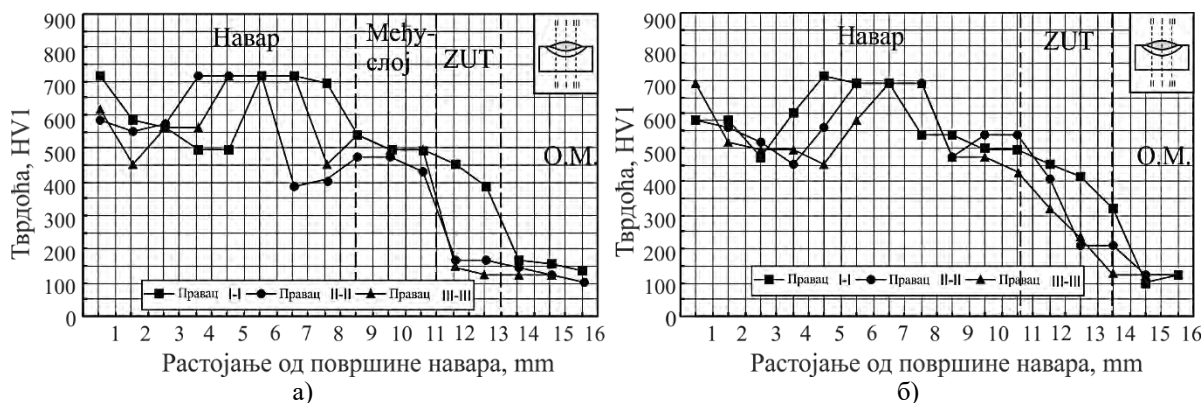
Слика 9.3.5 Расподела тврдоћа по пресеку трослојног наvara: а) O.M.- \check{C}0363 ; D.M. међуслоја - INOX B 18/8/6; D.M. наvara - ABRADUR 58; б) O.M.- \check{C}0363 ; D.M. наvara - ABRADUR 58
