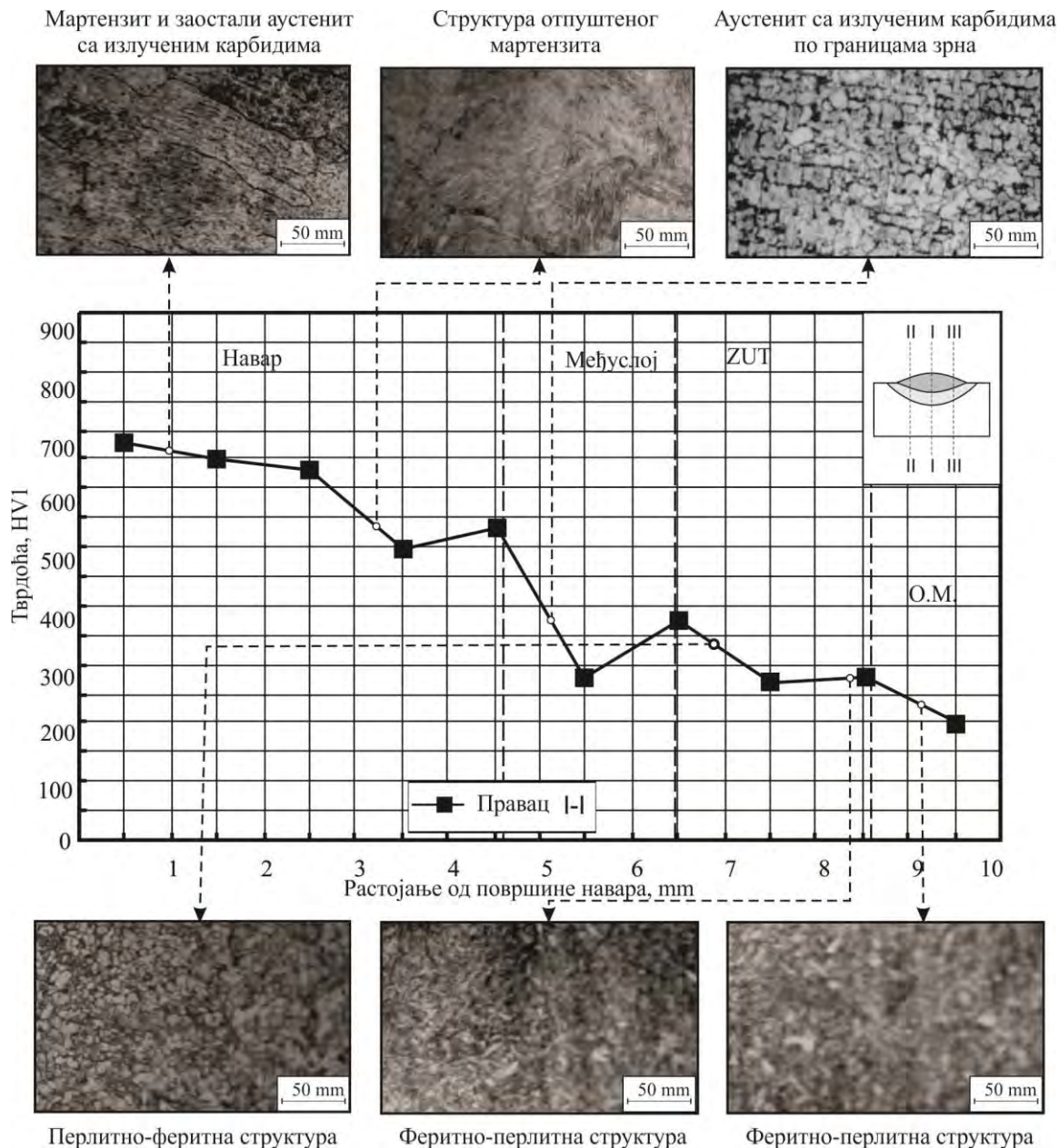
Слика 9.3.22 Микроструктура карактеристичних зона навареног споја: О.М. – \text{Č0363} ; Д.М. међуслоја – INOX В 18/8/6; Е.М. навара – E DUR 600
