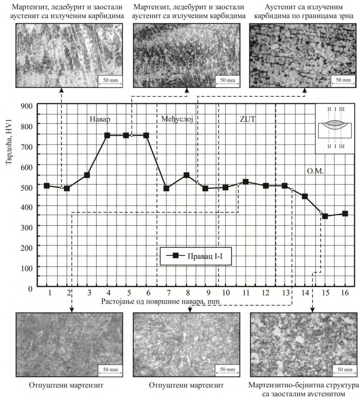
Слика 9.3.16 Микроструктура карактеристичних зона навареног споја: О.М. – \text{ČL3134} ; D.M. међуслоја - \text{INOX B 18/8/6} ; D.M. навара - \text{ABRADUR 58}
