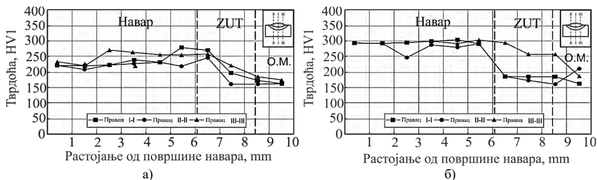
Слика 9.3.11 Расподела тврдоће по пресеку навара: а) O.M.- ČL3160, D.M. навар – E Mn 14; б) O.M.- ČL3460, D.M. навар – E Mn 17 Cr 13
