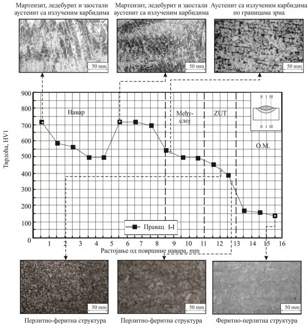
Слика 9.3.18 Микроструктура карактеристичних зона навареног споја: О.М. – \text{Č363} ; D.M. међуслоја - INOX B 18/8/6; D.M. наvara - ABRADUR 58
