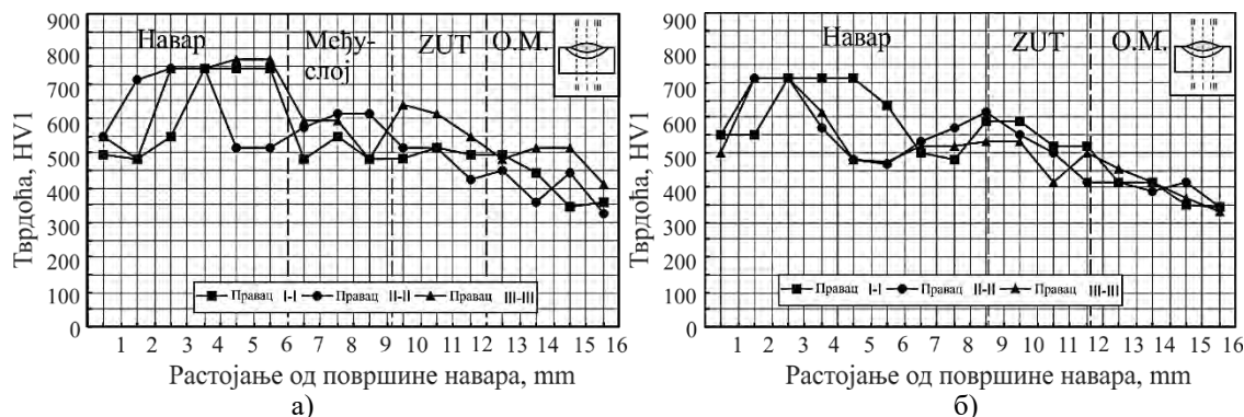
Слика 9.3.4 Расподела тврдоће по пресеку наvara: а) O.M. - \check{C}L3134 ; D.M. међуслоја - INOX B 18/8/6 D.M. наvara - ABRADUR 58; б) O.M. - \check{C}L3134 , D.M. наvara - ABRADUR 58
