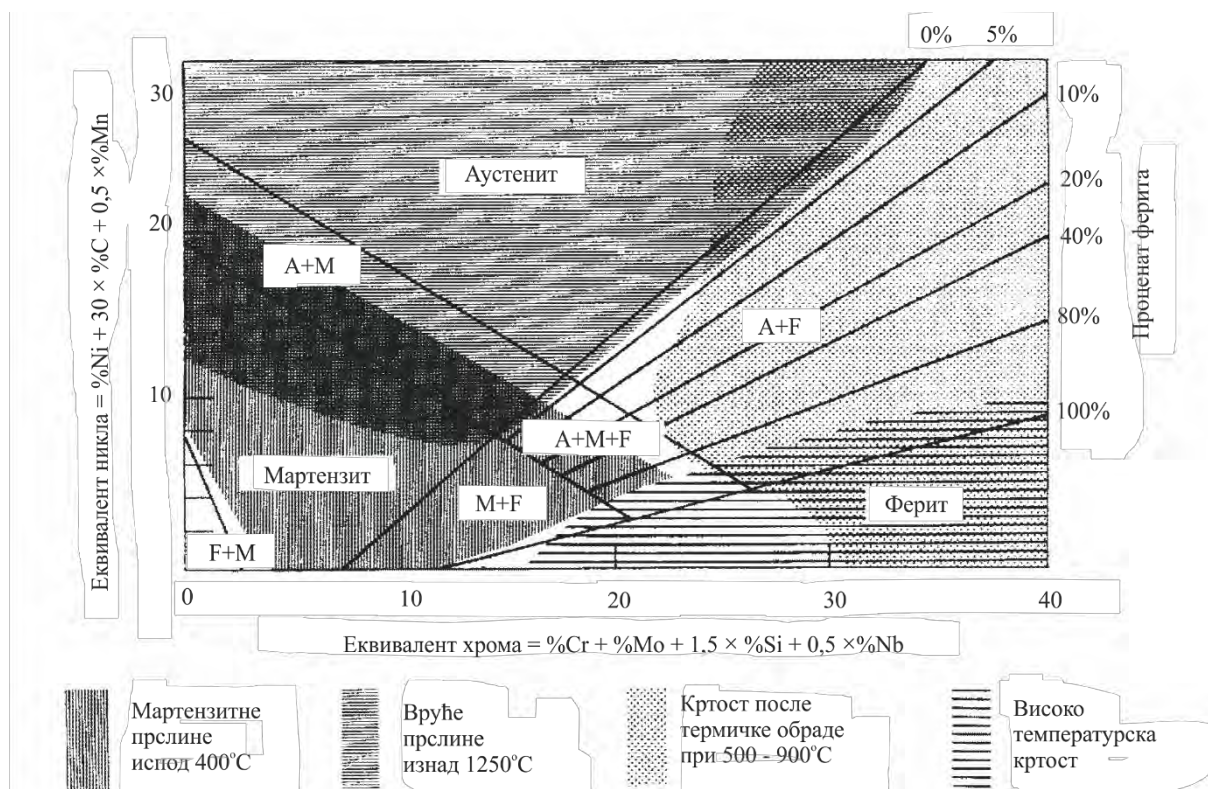
Слика 3.1 Локација грешки у зависности од структуре у Шефлеровом дијаграму [63,141]
