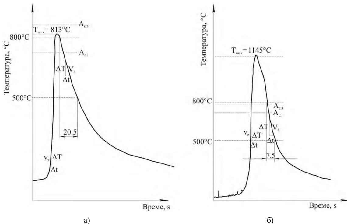
Слика 9.5.3 Температурски циклус ZUT-а при наваривању: а) Č0561 ( s=10\text{ mm} , x=3,5\text{ mm} , d_e=5\text{ mm} , T_p=96\text{ }^\circ\text{C} , q_l=16700\text{ J/cm} ); б) Č1530 ( s=20\text{ mm} , x=4\text{ mm} , d_e=4\text{ mm} , T_p=50\text{ }^\circ\text{C} , q_l=17900\text{ J/cm} ) [97]
