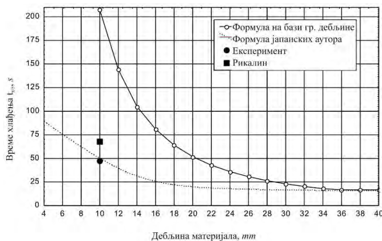
Слика 9.5.9 Упоредни резултати времена хлађења t_{8/5} за Ć0561 дебљине s = 10 mm, при наваривању: T_p = 62 °C, d_e = 5 mm, q_1 = 34017 J/cm [97]
