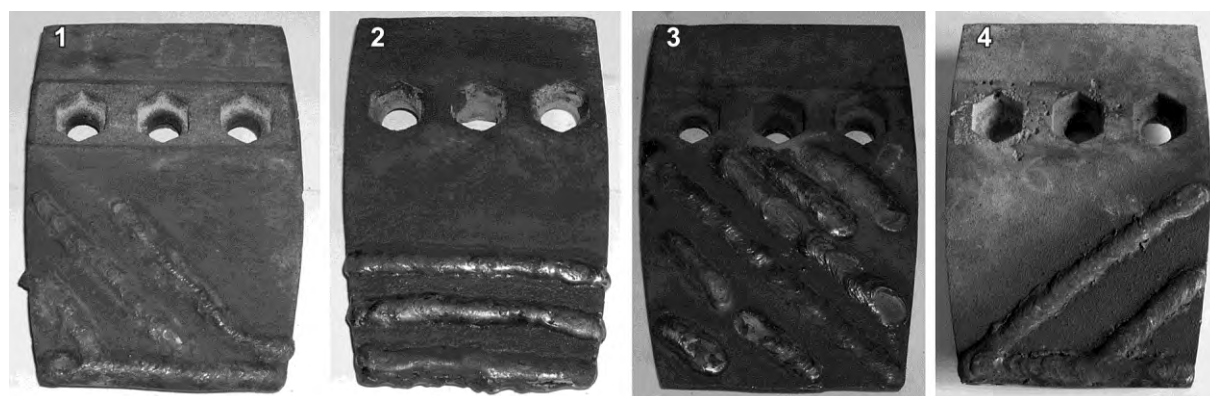
Слика 9.6.16 Изглед наварених узорка лопатица: 1-навар од D.М.-E DUR 600; 2,3-навар од D.М.-ABRADUR 58; 4-навар од D.М.-CrWC 600
