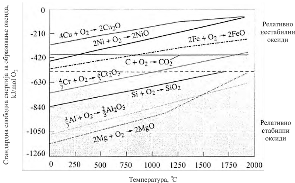
Слика 1.8 Стандардна слободна енергија за формирање неких оксида у функцији температуре (виша енергија – већа склоност ка оксидацији) [7,22]
