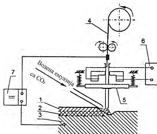
Слика 2.15 Модификације GMA наваривања: 1-навар, 2-зона топљења, 3-основни материјал, 4-електрода, 5-вibrator, 6-извор струје за напајање vibratorа, 7-извор струје [63,97,141]
