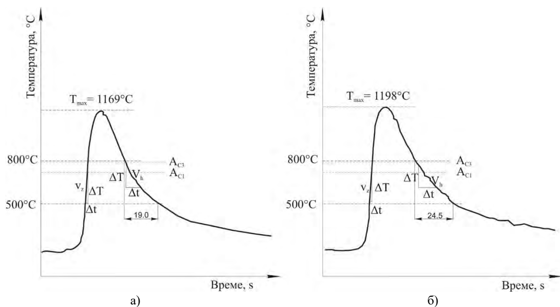
Слика 9.5.14 Температурски циклус ZUT-а при наваривању Č5742 дебљине s = 7,4 mm; електродом пречника d_e = 3,25 mm: а) наваривање ( T_p = 178^{\circ}\text{C} , v_z = 0,183 cm/s, q_l = 12568 J/cm); б) наваривање ( T_p = 180^{\circ}\text{C} , v_z = 0,150 cm/s, q_l = 15333 J/cm) [97]
