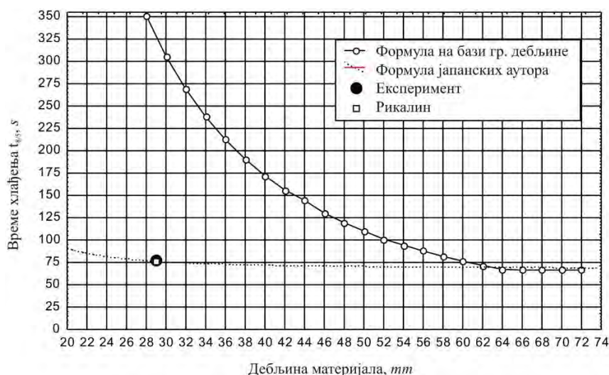
Слика 9.5.20 Упоредни резултати времена хлађења t_{8/5} за \text{Č5742} дебљине s = 29 mm, при наваривању: T_p = 355^\circ\text{C} , d_e = 5 mm, q_1 = 32738 J/cm [97]
