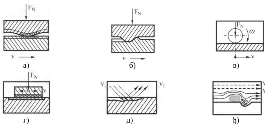
Слика 1.6 Схематски приказ основних врста хабања: а) адхезионо хабање, б) абразивно хабање, в) заморно хабање, г) вибрационо хабање, д) ерозионо хабање, њ) кавитационо хабање [14,141]
