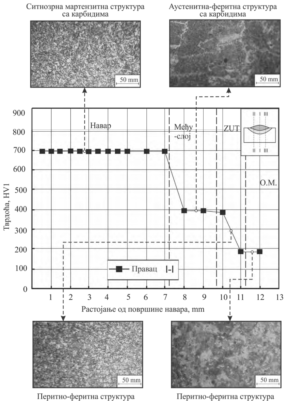
Слика 9.3.30 Микроструктура карактеристичних зона навареног споја: О.М. – \text{S0645} ; D.M. међуслоја – \text{FILTUB 12 B} ; D.M. навара – \text{FILTUB DUR 16}
