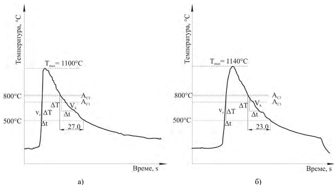
Слика 9.5.13 Температурски циклус ZUT-а при наваривању Č5742 дебљине s = 7,4 mm, електродом пречника d_e = 3,25 mm: а) наваривање ( T_p = 180^{\circ}\text{C} , v_z = 0,208 cm/s, q_l = 11058 J/cm); б) наваривање ( T_p = 178^{\circ}\text{C} , v_z = 0,190 cm/s, q_l = 12105 J/cm) [97]
