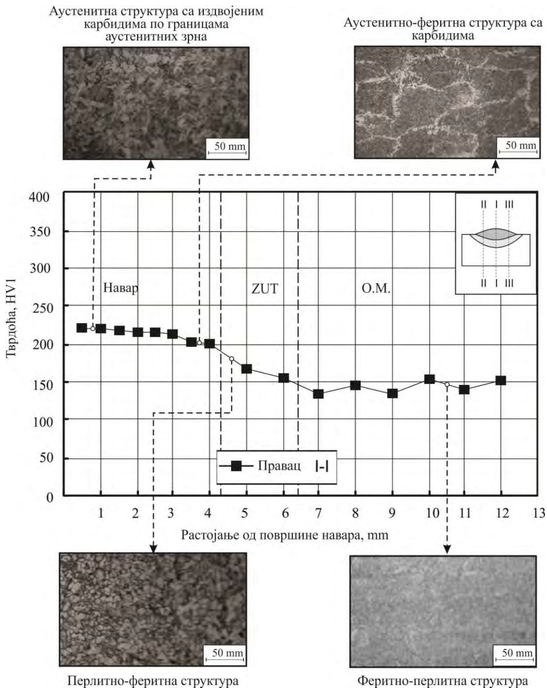
Слика 9.3.28 Микроструктура карактеристичних зона навареног споја: О.М. – \text{Č0363} ; Д.М. навара – FILTUB 12 В
