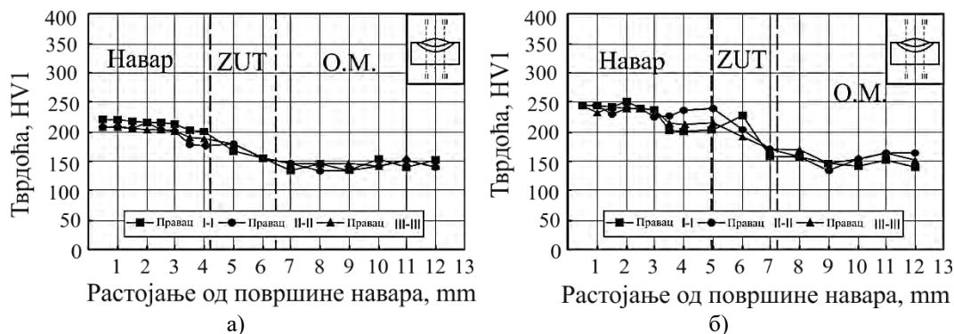
Слика 9.3.12 Расподела тврдоће по пресеку навара: а) O.M. – Č0363, D.M. навар - FILTUB 12 B; б) O.M. – Č0645, D.M. навар - FILTUB 12 B
