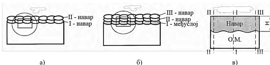
Слика 9.4.9 Начин припреме блокова за триболошка испитивања: а) сечење блока из двослојног наvara, б) сечење блока из трослојног наvara, в) изглед блока
