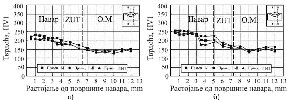
Слика 9.3.13 Распдела тврдоће по пресеку навара: а) O.M.-Č0363, D.M. навара – FILTUB 12 B; б) O.M.-Č0645, D.M. навара – FILTUB 12 B
