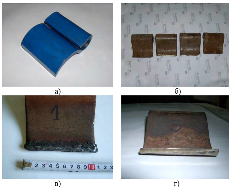
Слика 9.6.31 Изглед ножева уређаја за равнање терена: а) нов нож, б) похабани ножеви, в) наварени нож, г) наоштрен нож
