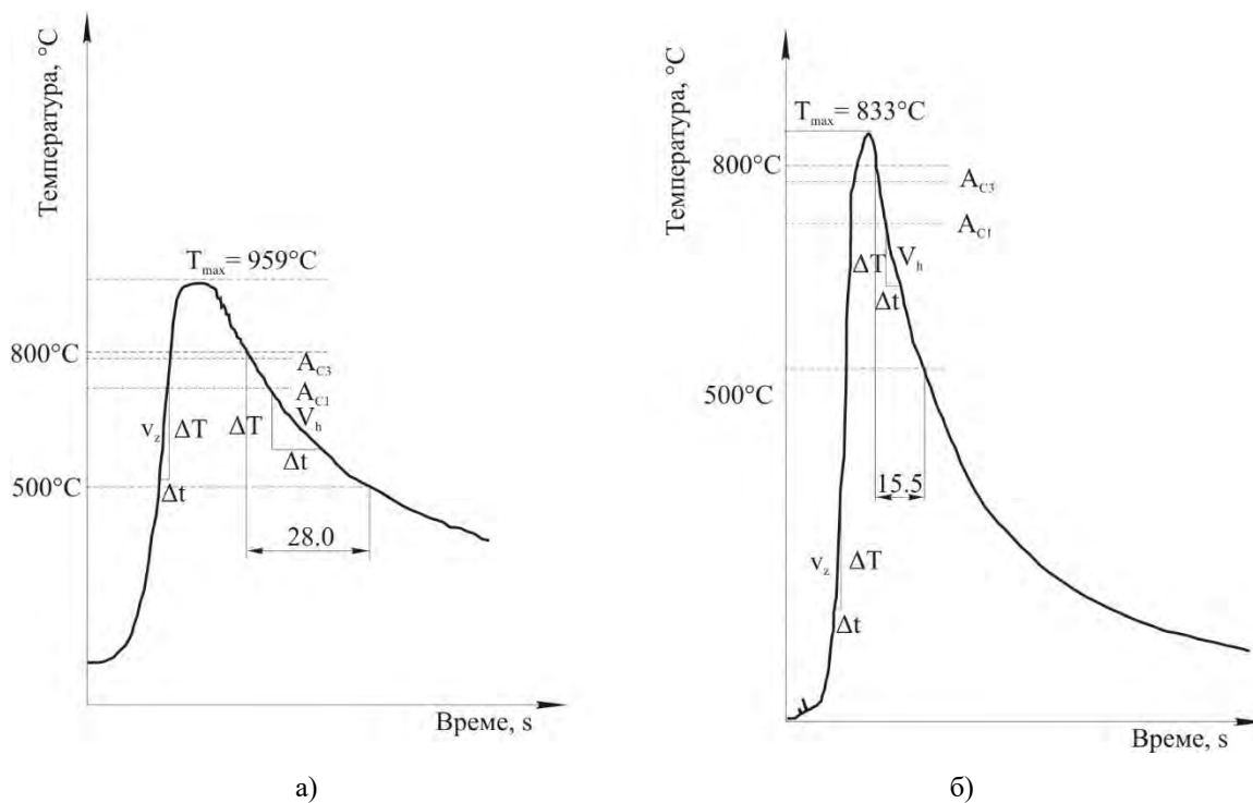
Слика 9.5.4 Температурски циклус ZUT-а при наваривању: а) Č1530 ( s=20\text{ mm} , x=4\text{ mm} , d_e=5\text{ mm} , T_p=100\text{ }^\circ\text{C} , q_l=35800\text{ J/cm} ); б) Č1531 ( s=10\text{ mm} , x=4\text{ mm} , d_e=4\text{ mm} , T_p=20\text{ }^\circ\text{C} , q_l=18200\text{ J/cm} ) [97]
