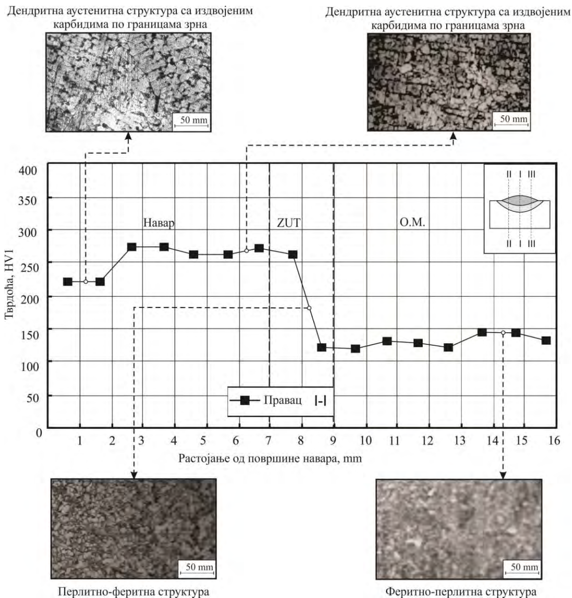
Слика 9.3.26 Микроструктура карактеристичних зона навареног споја: О.М. – \check{C}0363 ; D.M. навара – E Mn 14
