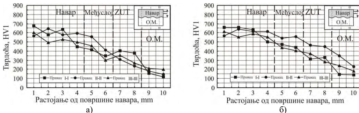
Слика 9.4.12 Расподела тврдоће код блокова припремљених за триболошка испитивања: а) О.М.-Č0363, D.M. међуслоја - INOX B 18/8/6, D.M. наvara – CrWC 600; б) О.М.-Č0363, D.M. међуслоја - INOX B 18/8/6, D.M. - наvara E DUR 600
