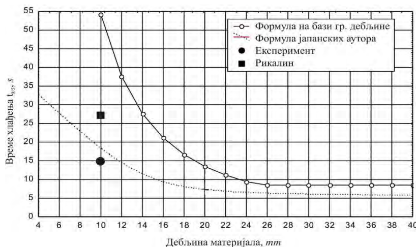
Слика 9.5.8 Упоредни резултати времена хлађења t_{8/5} за \check{C}1531 дебљине s=10\text{ mm} , при наваривању: T_p = 36^\circ\text{C} , d_e = 4\text{ mm} , q_l = 19413\text{ J/cm} [97]
