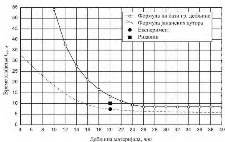
Слика 9.5.10 Упоредни резултати времена хлађења t_{8/5} за Ć1530 дебљине s = 20 mm, при наваривању: T_p = 50 °C, d_e = 4 mm, q_1 = 17975 J/cm [97]
