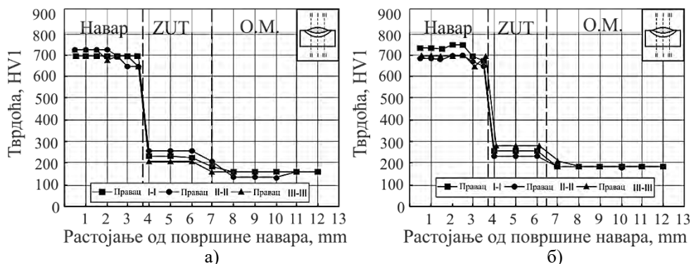
Слика 9.3.15 Распдела тврдоће по пресеку двослојног навара: а) O.M.-Č0363, D.M. навара - FILTUB DUR 16; б) O.M.-Č0645, D.M. навара - FILTUB DUR 16
