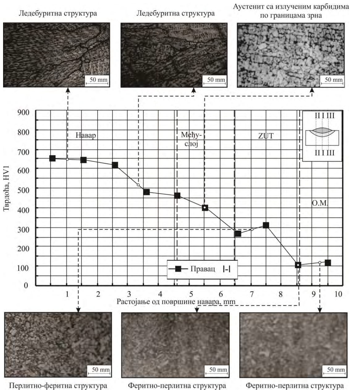
Слика 9.3.20 Микроструктура карактеристичних зона навареног споја: О.М. – \check{C}0363 ; D.M. међуслоја - INOX B 18/8/6; D.M. навара – CrWC 600
